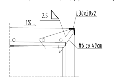
Detal zabezpieczenia krawędzi płyty fundamentowej
